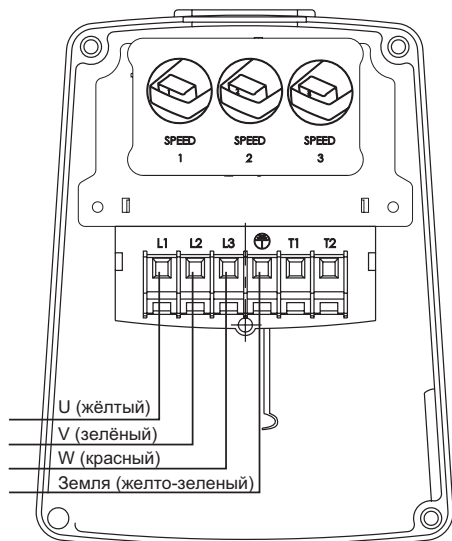
Рис. 22 Модуль переключения частоты вращения
