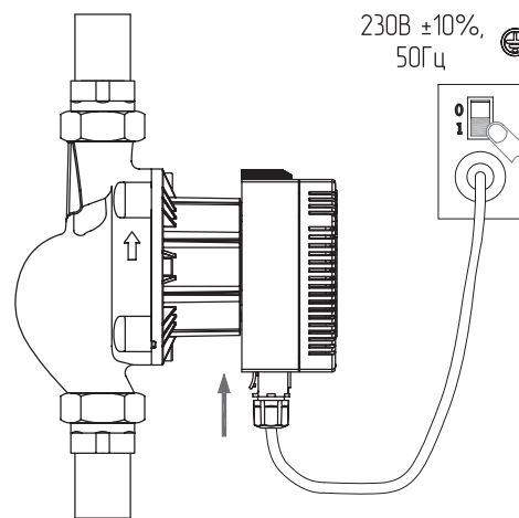
Рис. 40 Электроподключение насоса
