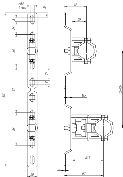
Кронштейн VG-900002
