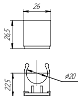
Клипса маркировочная VG-900004
