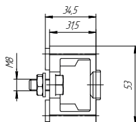
Удлинитель кронштейна VG-900003
