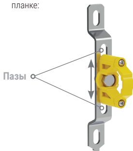
Рисунок 6. Пазы для регулирования межосевого расстояния.
