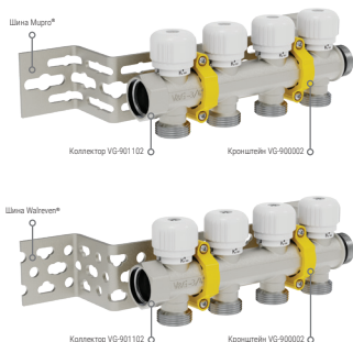
Рисунок 10. Установка коллектора на монтажные шины других производителей
