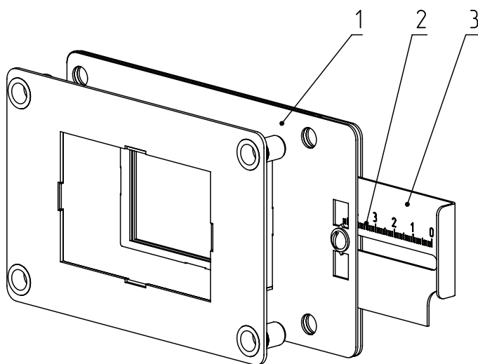
Рис.14 Заслонка вентилятора
