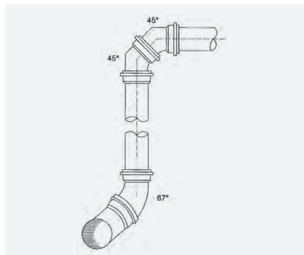
РИС. 12. ПРИМЕР ВЕРТИКАЛЬНОГО ПОДКЛЮЧЕНИЯ К ГЛАВНОМУ КАНАЛИЗАЦИОННОМУ КАНАЛУ
