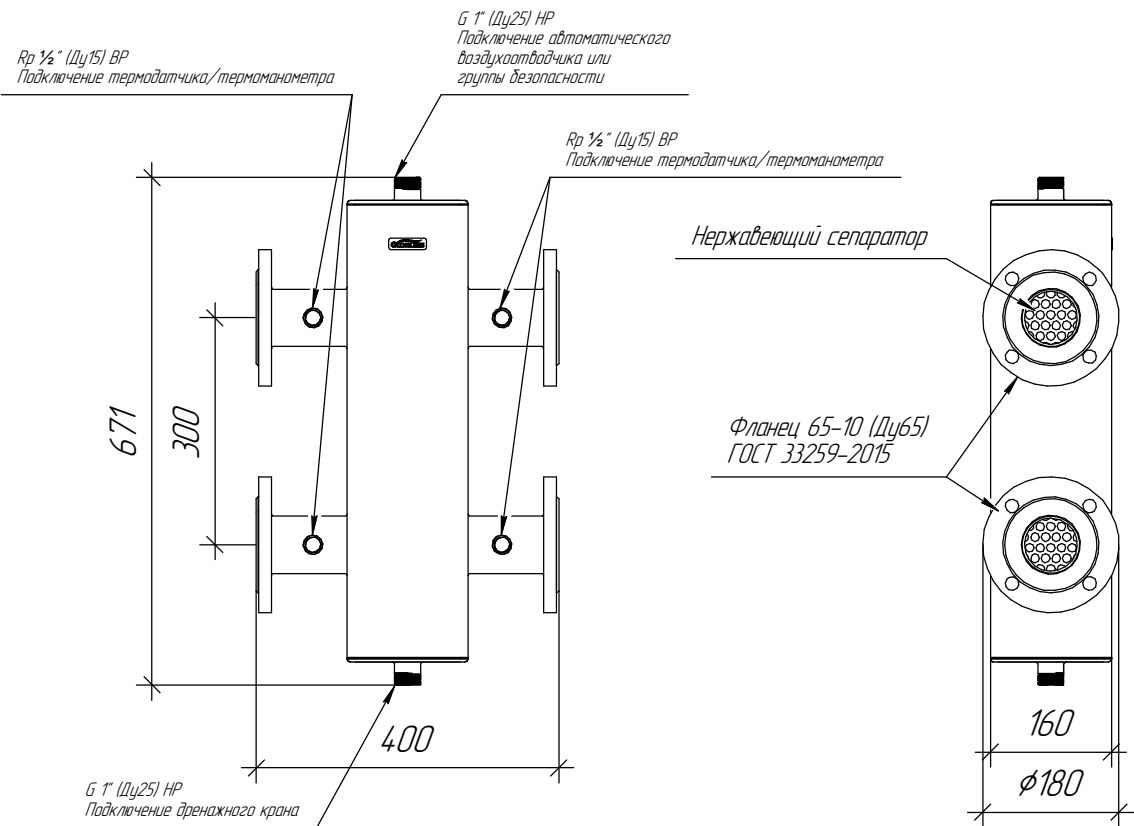
Монтажные размеры
