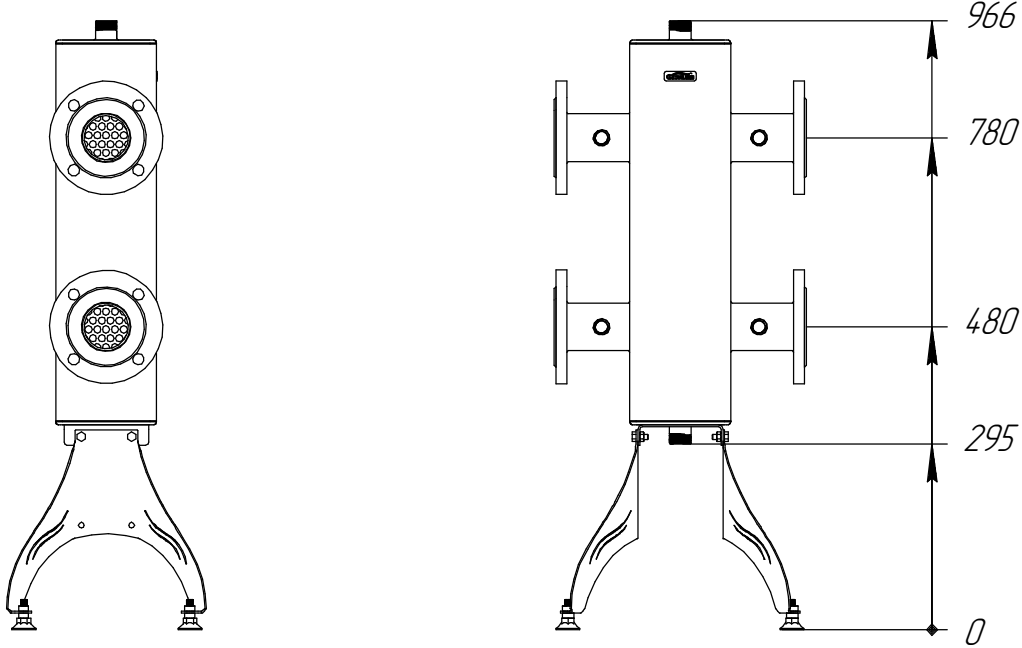
Монтажные размеры
