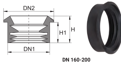
DN 160-200
